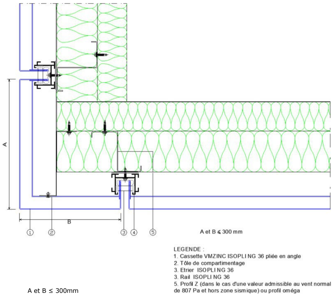
Figure 31 - Angle sortant sur plateaux
