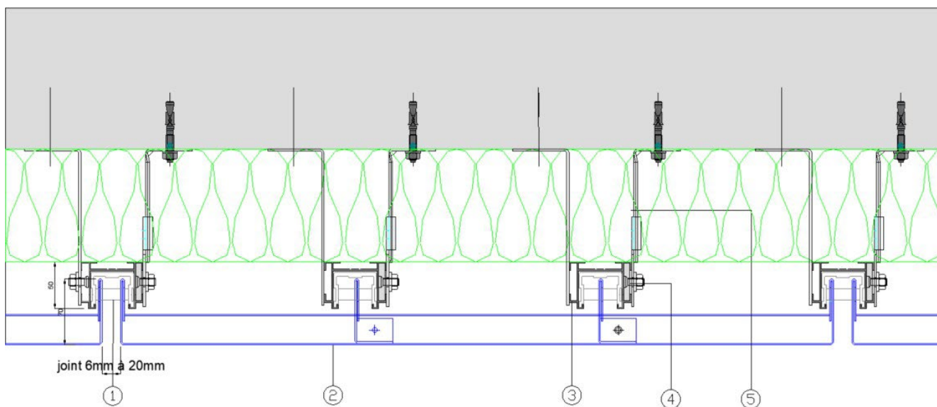
Figure 3b Joint vertical (coupe horizontale) avec rails dilatants
