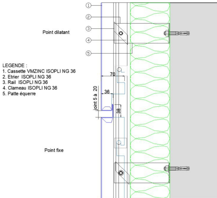
Figure 4b – Joint horizontal (coupe verticale) sur cassettes horizontales avec raidisseurs, exemple avec rails ISOPLING de 3 m maximum
