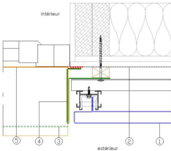
Coupe sur tableau , situation a, b, c
