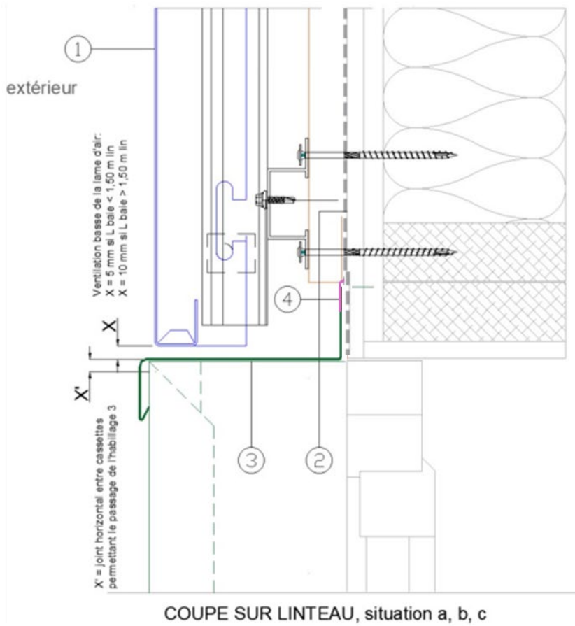
Figure 23d – Linteau sur COB et CLT, linteau au nu extérieur
