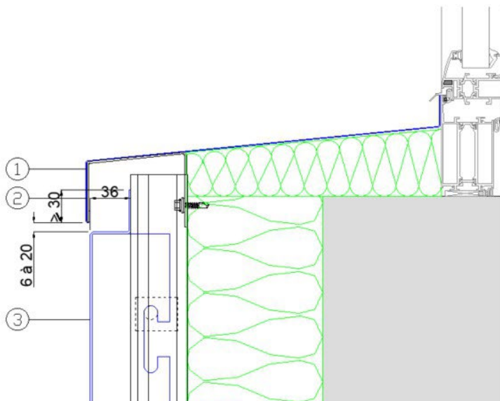
Figure 14 - Appui de baie
