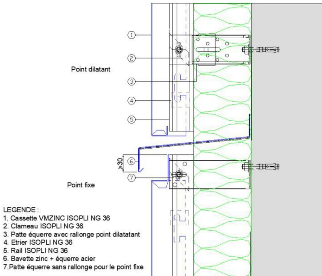
Figure 9- Compartimentage horizontal de la lame d'air
