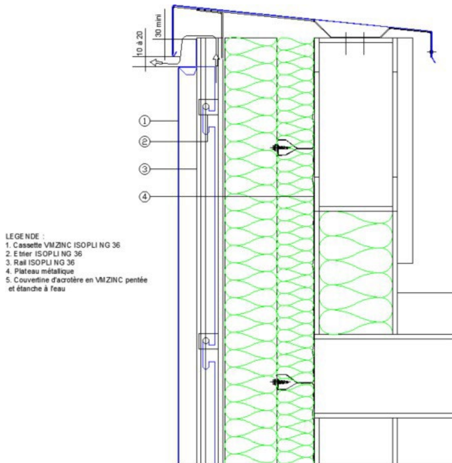
Figure 29- Acrotère sur plateaux
