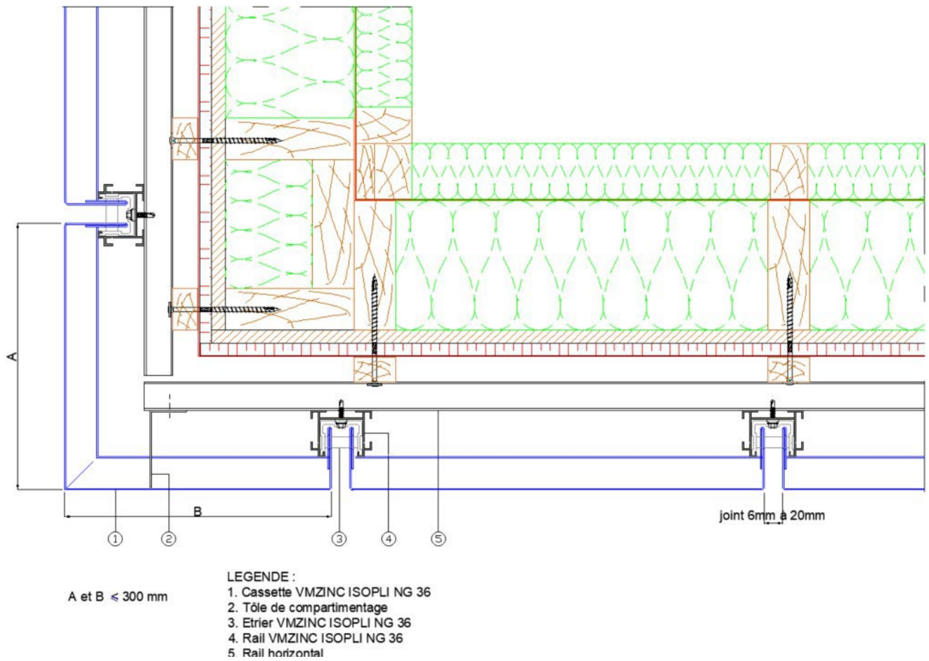
Figure 20 – Angle sortant sur COB et CLT
