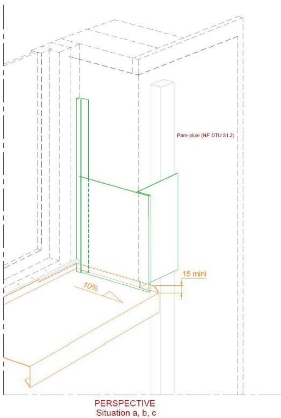
Figure 23c – Dispositions particulières du traitement des baies sur COB et CLT Appui de baie et tableau (Menuiserie en tunnel intérieur)
