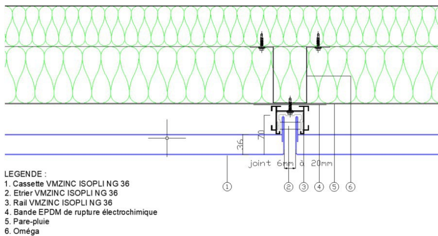
Figure 25b – coupe horizontale sur plateaux avec profils oméga (exigé en zones sismiques ou au-delà d'une résistance admissible au vent normal de 807 Pa)
