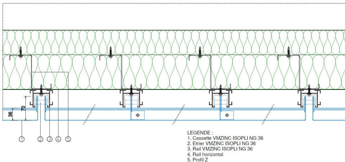
Figure 26 : Cassettes horizontales avec raidisseurs sur plateaux. Coupe horizontale
