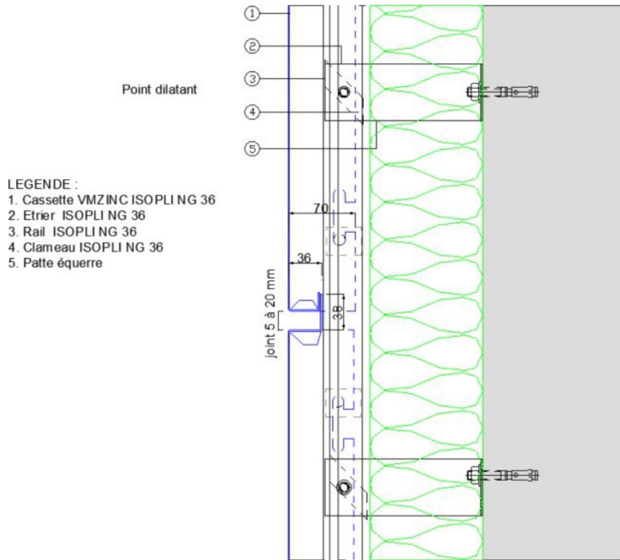
Figure 4 – Joint horizontal (coupe verticale) avec rails ISOPLING de 3 m maximum
