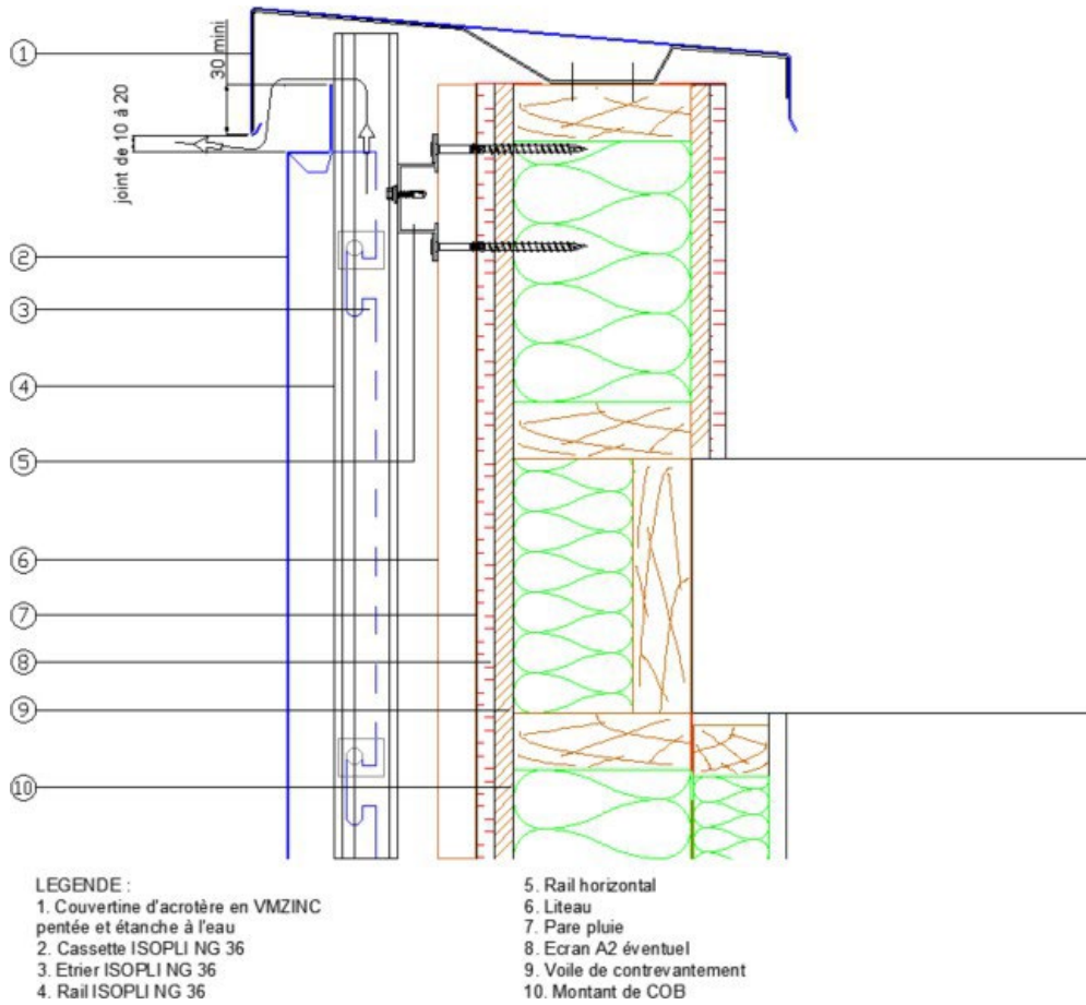
Figure 18 – Arrêt sur acrotère sur COB et CLT
