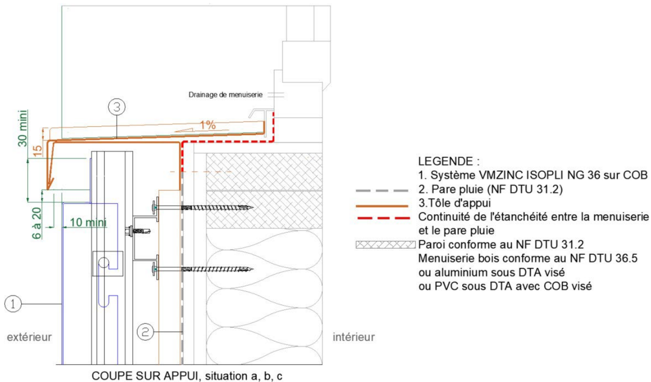
Figure 23b – Appui sur COB et CLT avec menuiserie au nu intérieur
