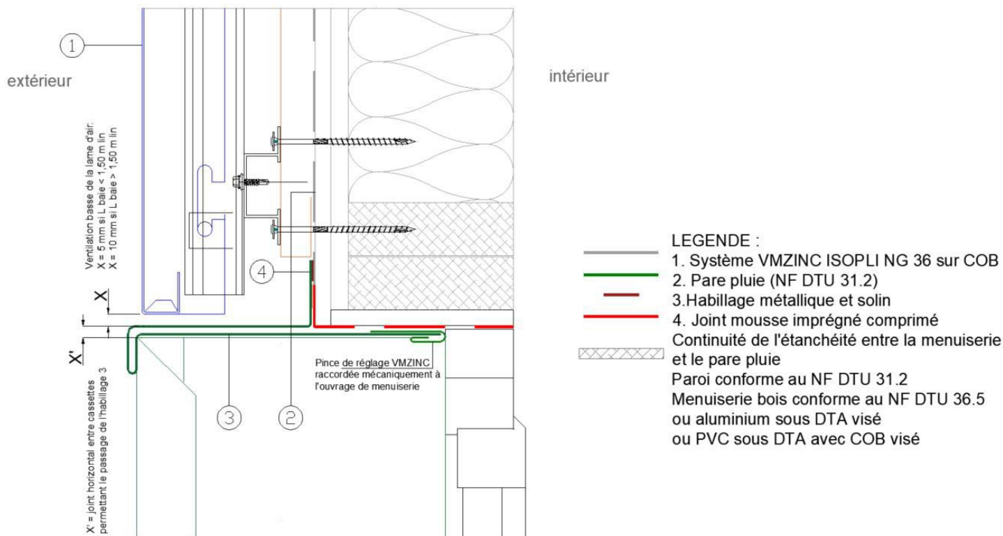
Figure 23a – Linteau sur COB et CLT avec menuiserie au nu intérieur
