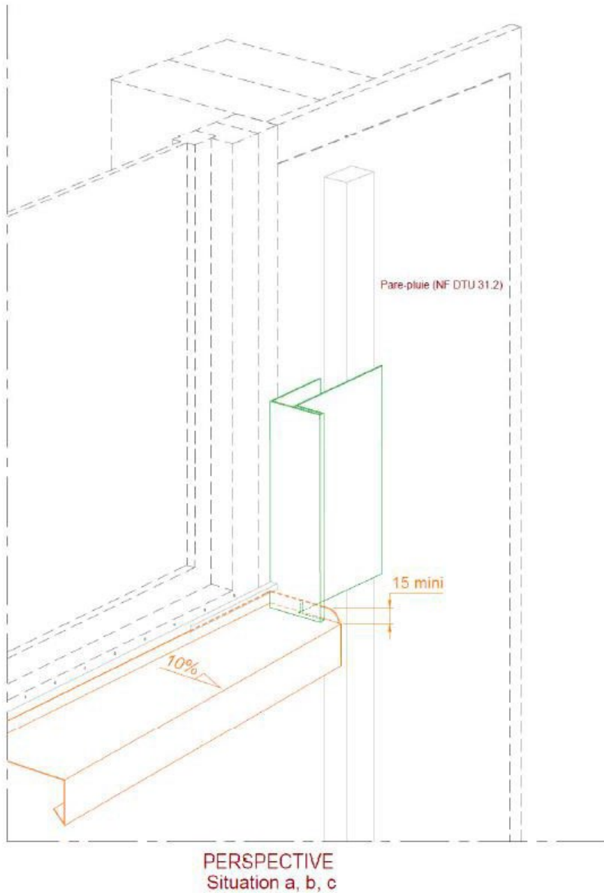
Figure 23g– Dispositions particulières du traitement des baies Bande d'appui et tableaux (Menuiserie en tunnel extérieur)
