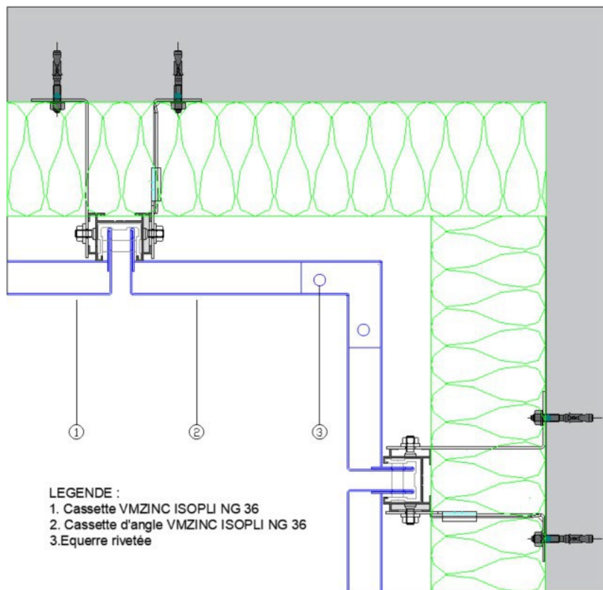
Figure 7b angle rentrant avec cassette d'angle
