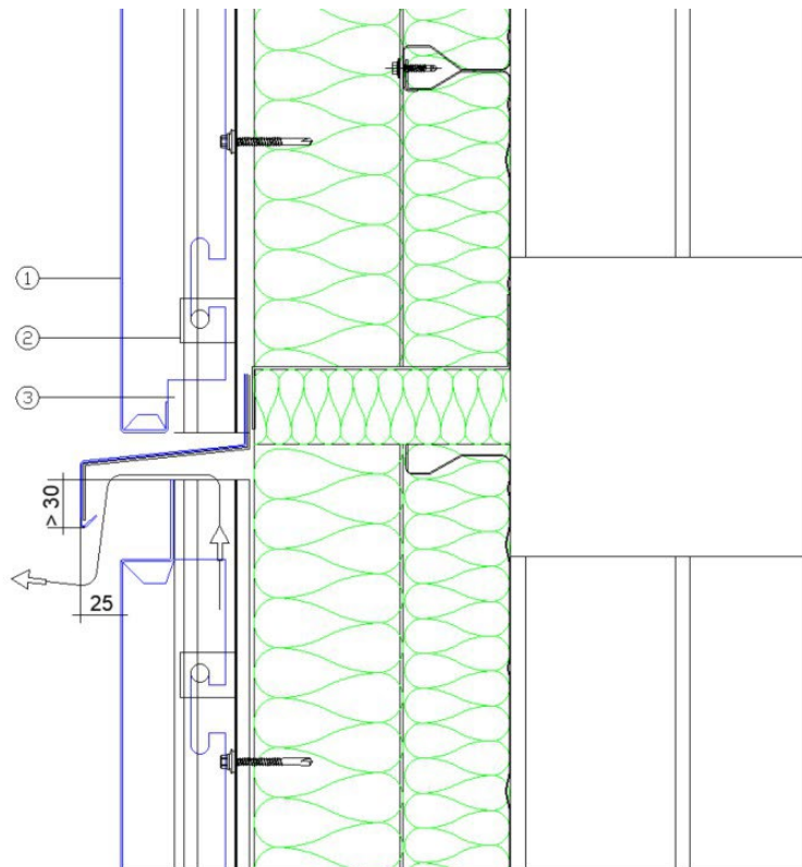
Figure 28 – Fractionnement horizontal de la lame d'air et recouvrement du pare pluie tous les 3 m sur plateaux
