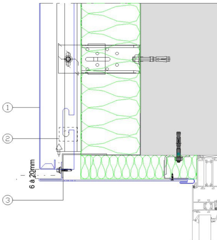
Figure 13 - Linteau de baie
