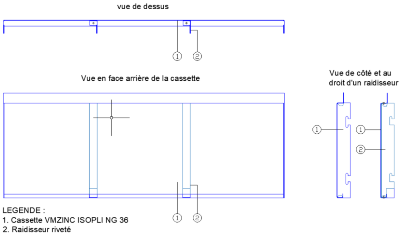
Figure 1e - Cassette ISOPLI NG 36 avec raidisseur
