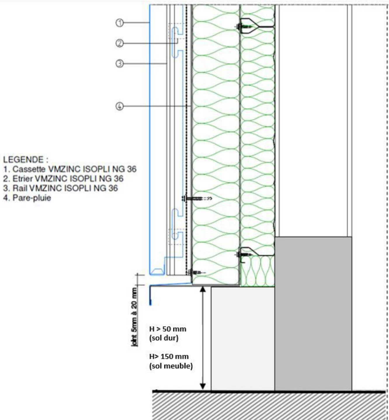
Figure 32 – Départ de bardage sur plateaux
