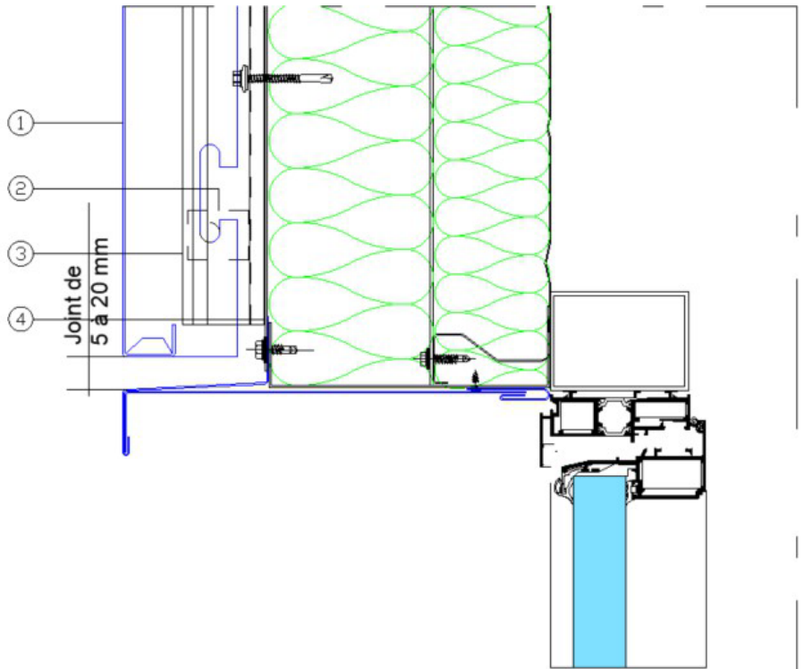
Figure 33- Linteau sur plateaux
