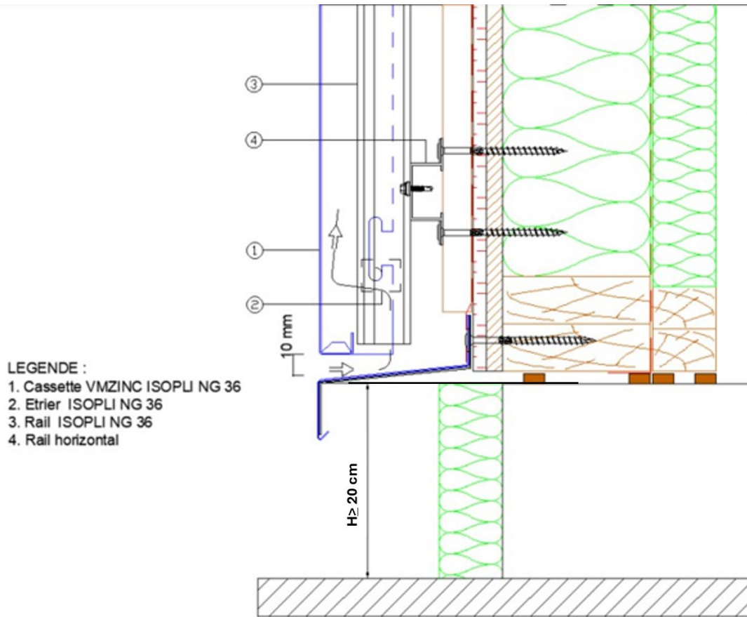
Figure 21 – Départ de bardage sur COB-et CLT
