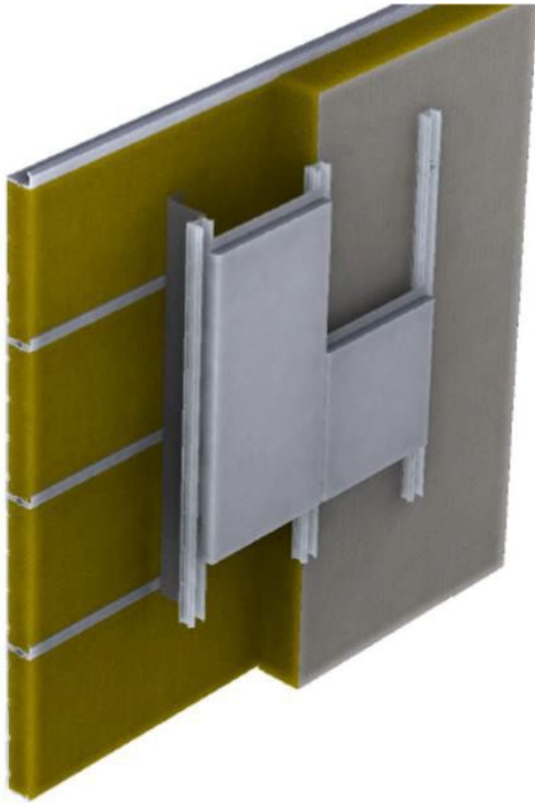
Ecarteurs réalisés avec des profils Z Sous réserve du respect des prescriptions indiqués au §1.4.3.
