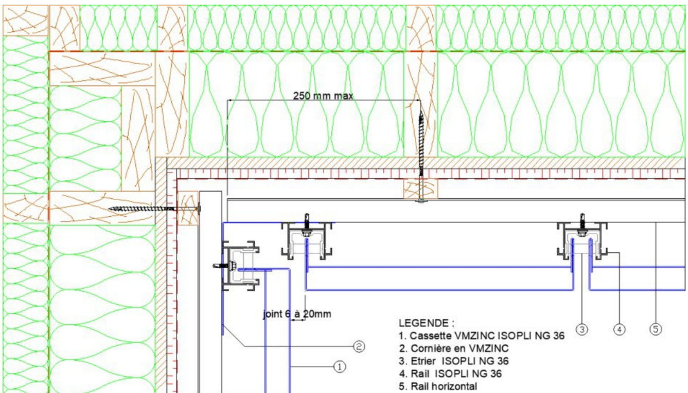
Figure 19 – Angle rentrant sur COB et CLT
