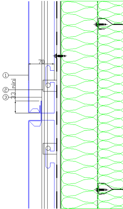
Figure 27 - Coupe verticale sur plateaux
