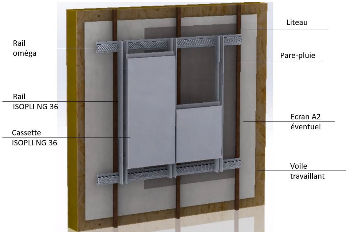
Figure 1b – Système ISOPLI NG 36 sur COB ou CLT
