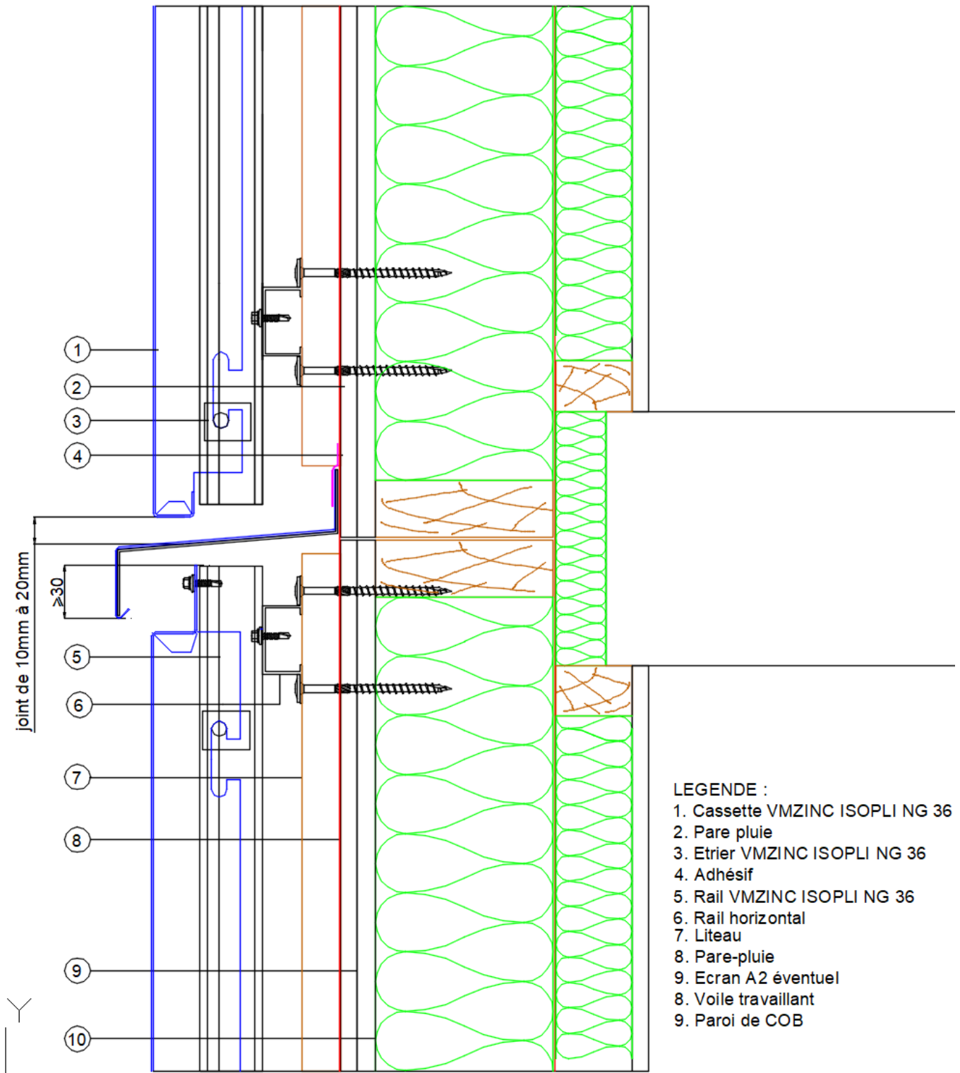
Figure 17 - Fractionnement horizontal de la lame d'air sur COB et CLT
