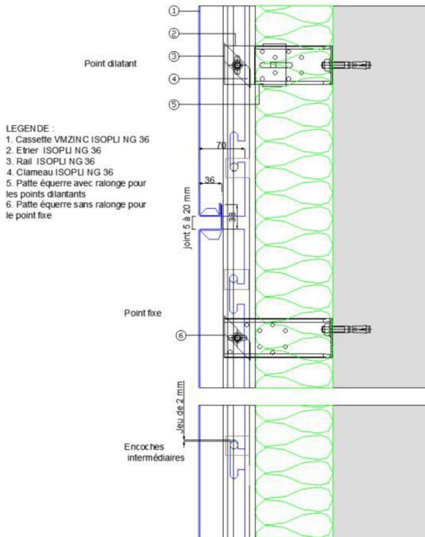
Figure 4c - Joint horizontal (coupe verticale) avec rails ISOPLI NG dilatants de 3 à 6 m
