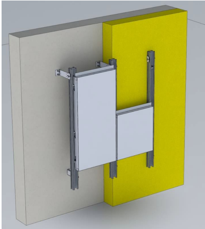
Figure 1a – Système ISOPLING 36 sur Maçonnerie
