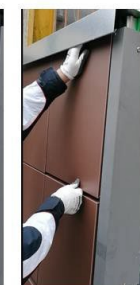
7. Pose de la cassette de remplacement
