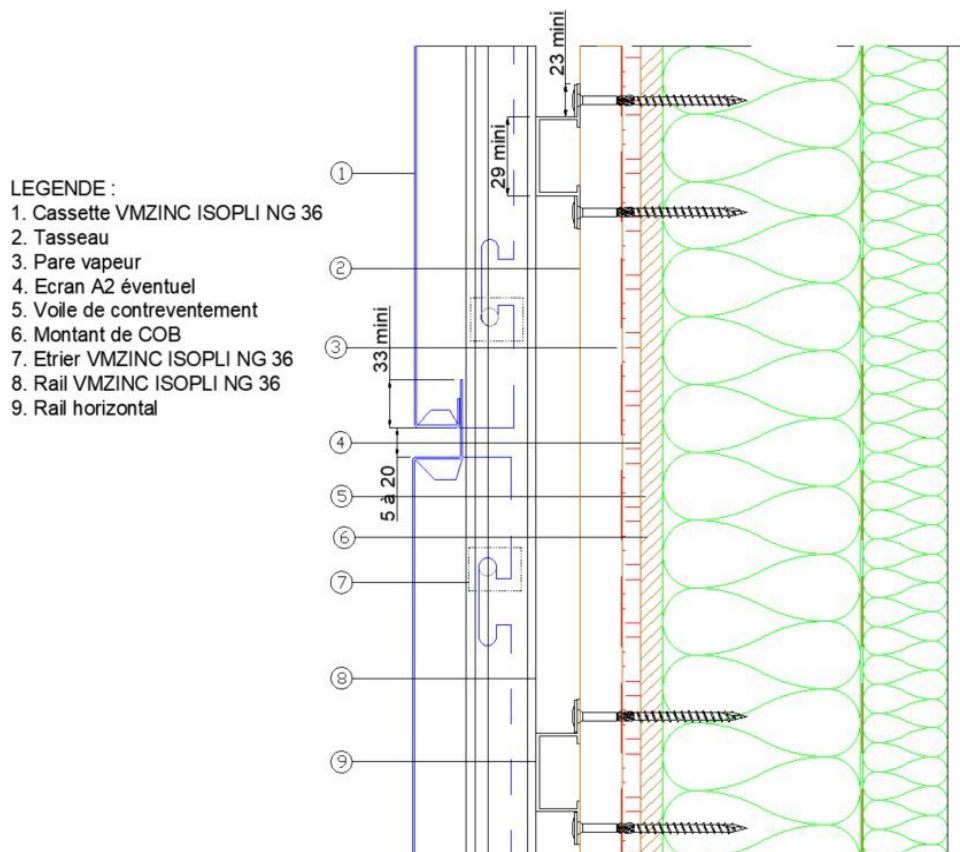
Figure 16 - Coupe verticale sur COB et CL
