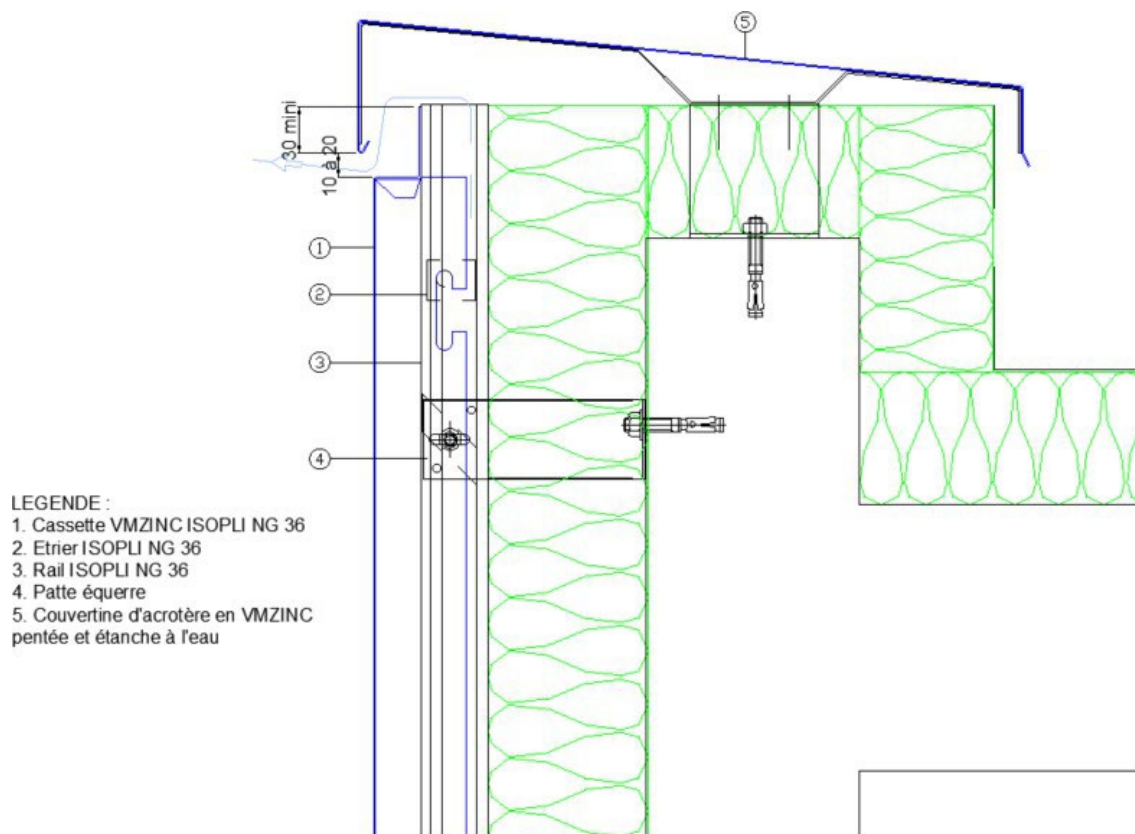
Figure 5 - Arrêt sur acrotère
