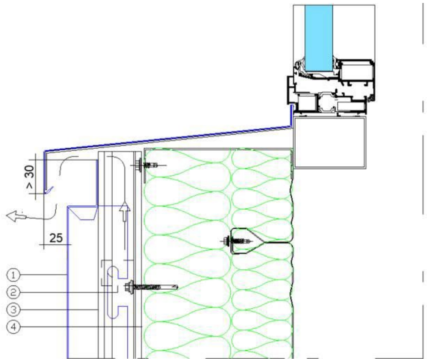
Figure 34 – Appui de baie sur plateaux
