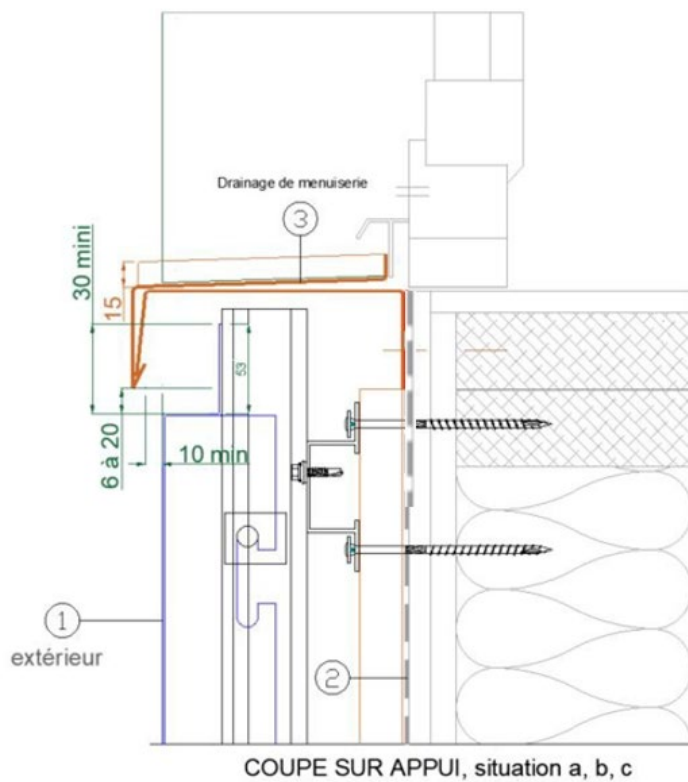
Figure 23e– Appui sur COB et CLT, Appui au nu extérieur
