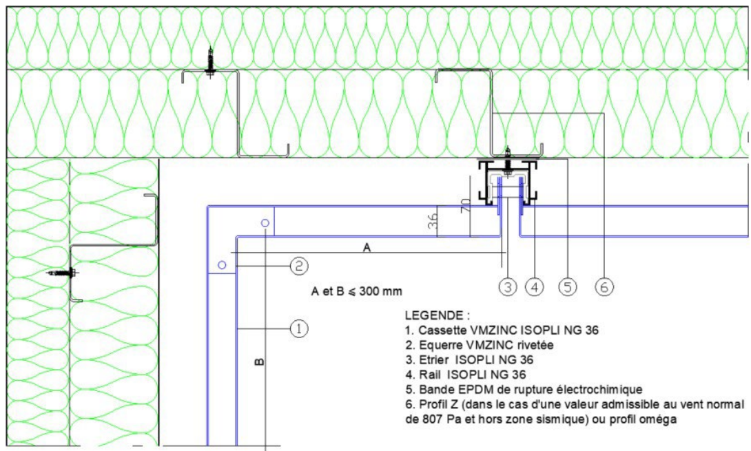
Figure 30b - Angle rentrant sur plateaux avec cassette d'angle rentrant
