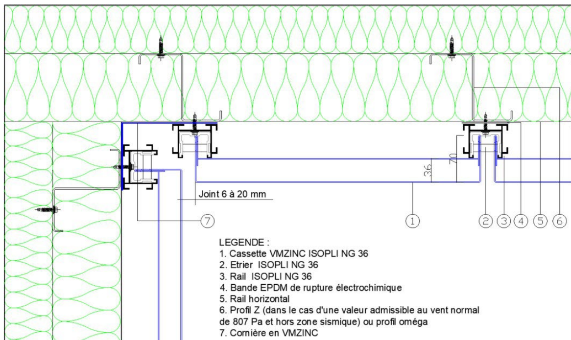
Figure 30 - Angle rentrant sur plateaux
