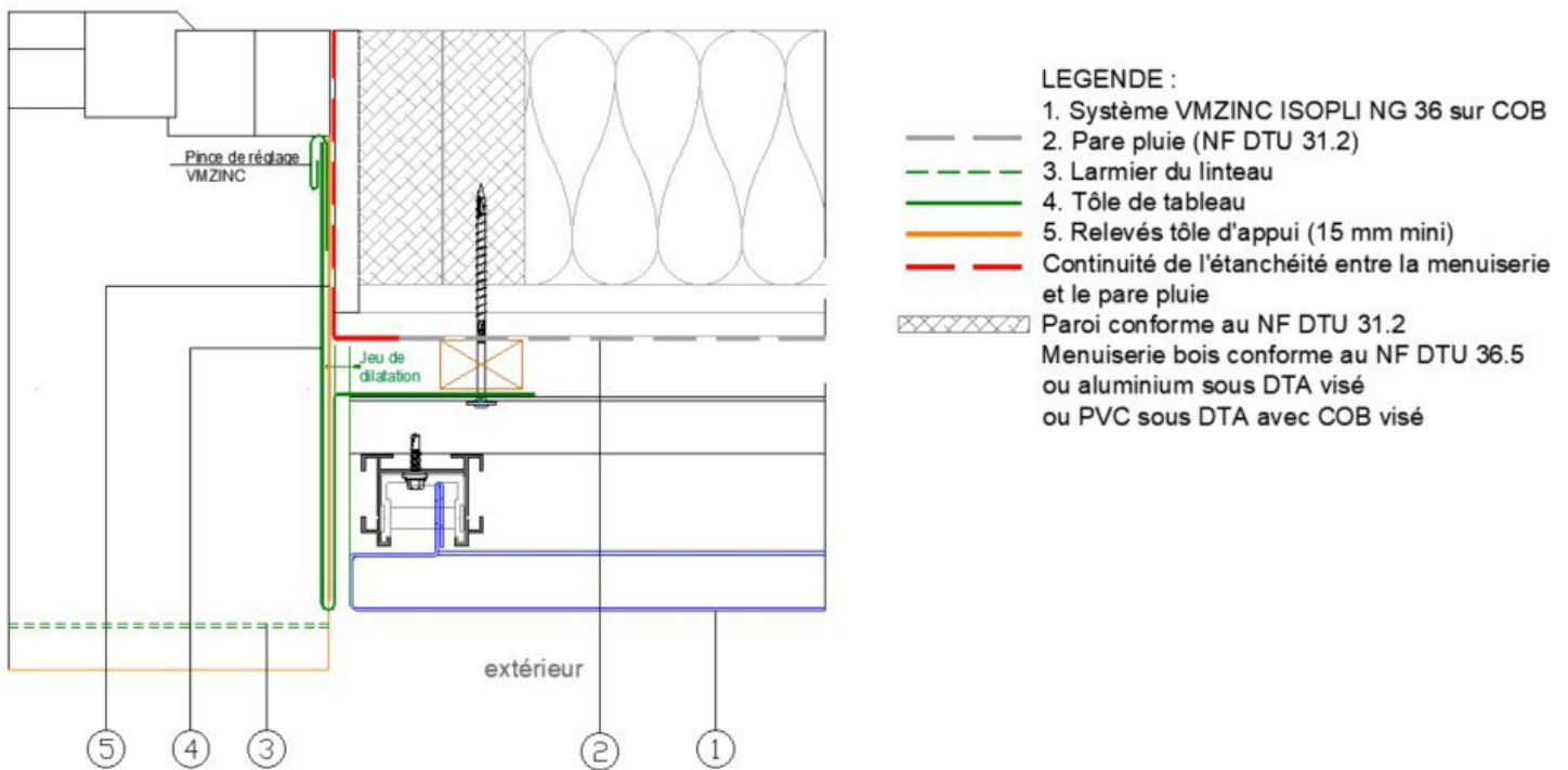
Coupe sur tableau , situation a, b, c
