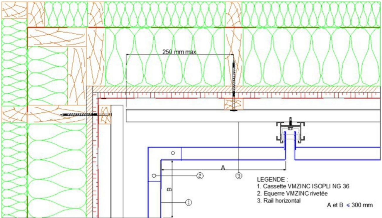
Figure 19b – Angle rentrant sur COB et CLT avec cassette d’angle rentrant
