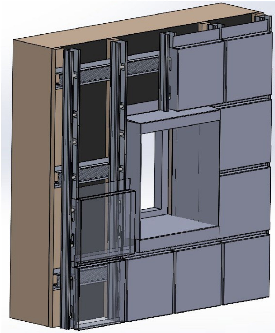
Figure 23c'– Dispositions particulières du traitement des baies sur COB et CLT Appui de baie et tableau (Menuiserie en tunnel intérieur)
