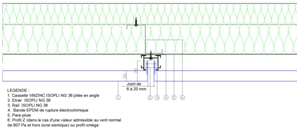
Figure 25 - Coupe horizontale sur plateaux
